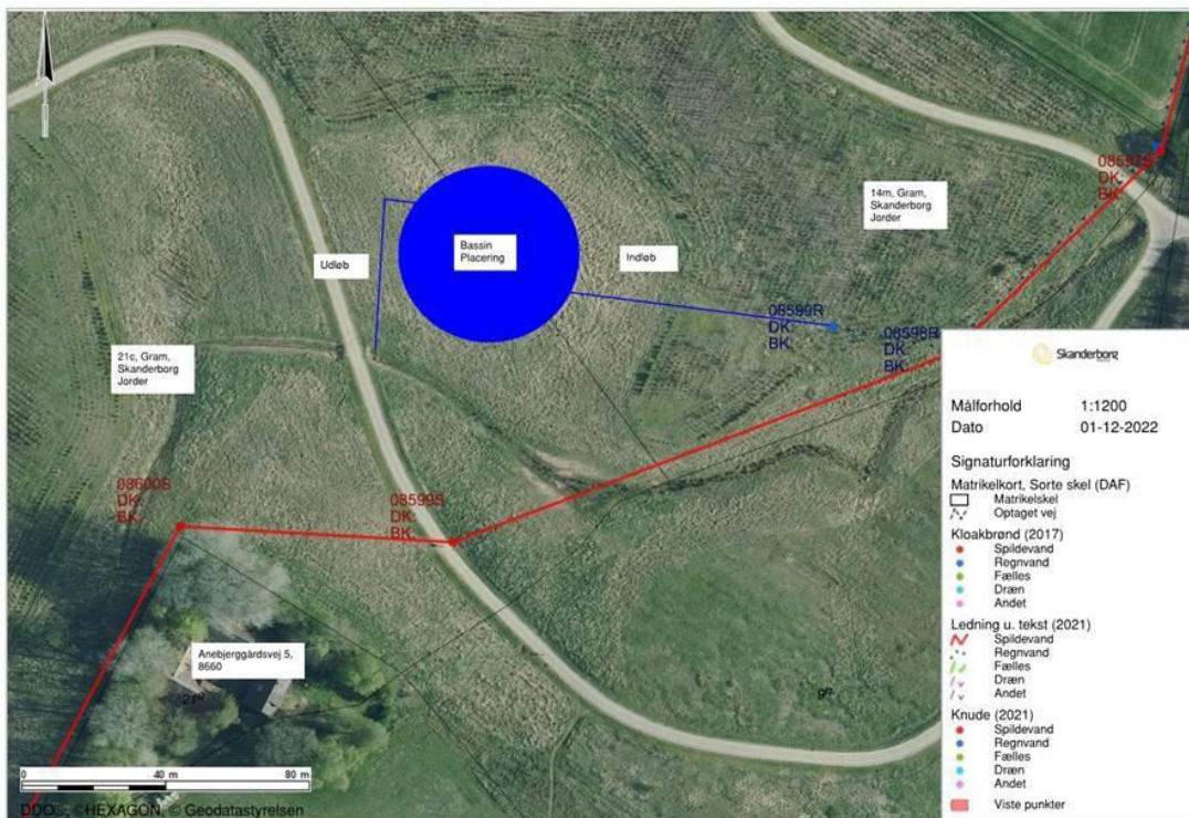
Figur 5 Plan bassin B600, men angivelse af ind- og udløb
